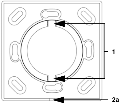
Abb. 2 Frontal-Ansicht
